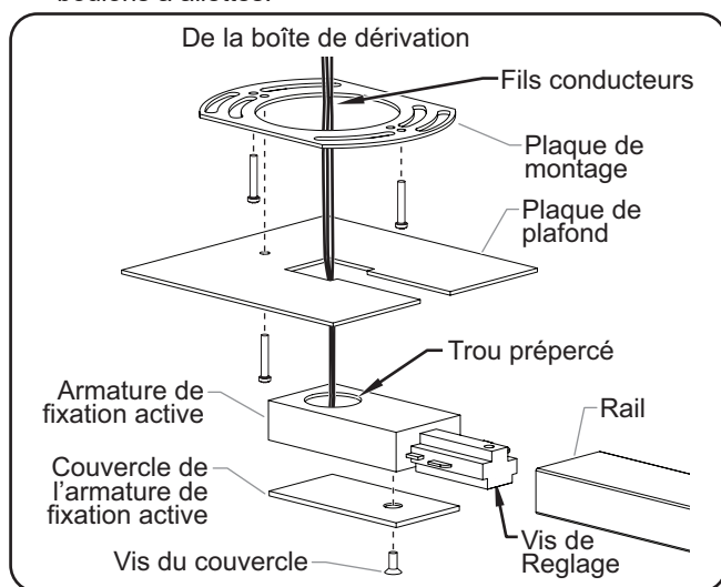
Installation du rail
