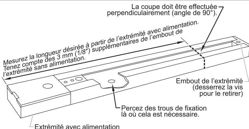
Coupe du rail à une longueur spécifique
